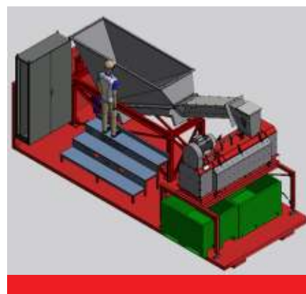
Mavitec Paddle Depacker Model S come soluzione containerizzata con un ingombro ridotto.
