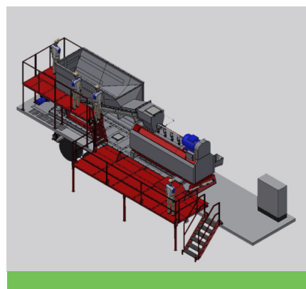
Лопастной распаковщик на колесах: мобильная прокатная единица для тестирования вашего сырья на вашем заводе.
