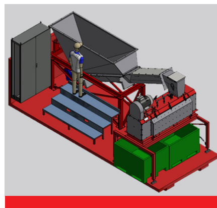
Лопастной Распаковщик модель S от Мавитек в виде контейнерного решения с небольшой занимаемой площадью
